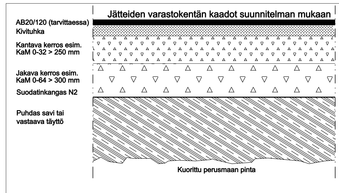
Rakenneleikkaus jätteiden varastokentästä 1:20
