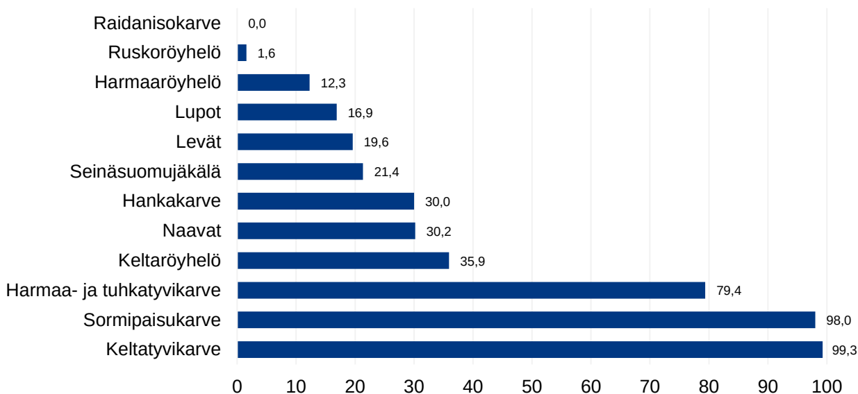
Kuva 4-9. Männyn runkojäkäläien prosentuaalinen esiintymistiheys tutkimusrungoilla 2022 (n = 960).
