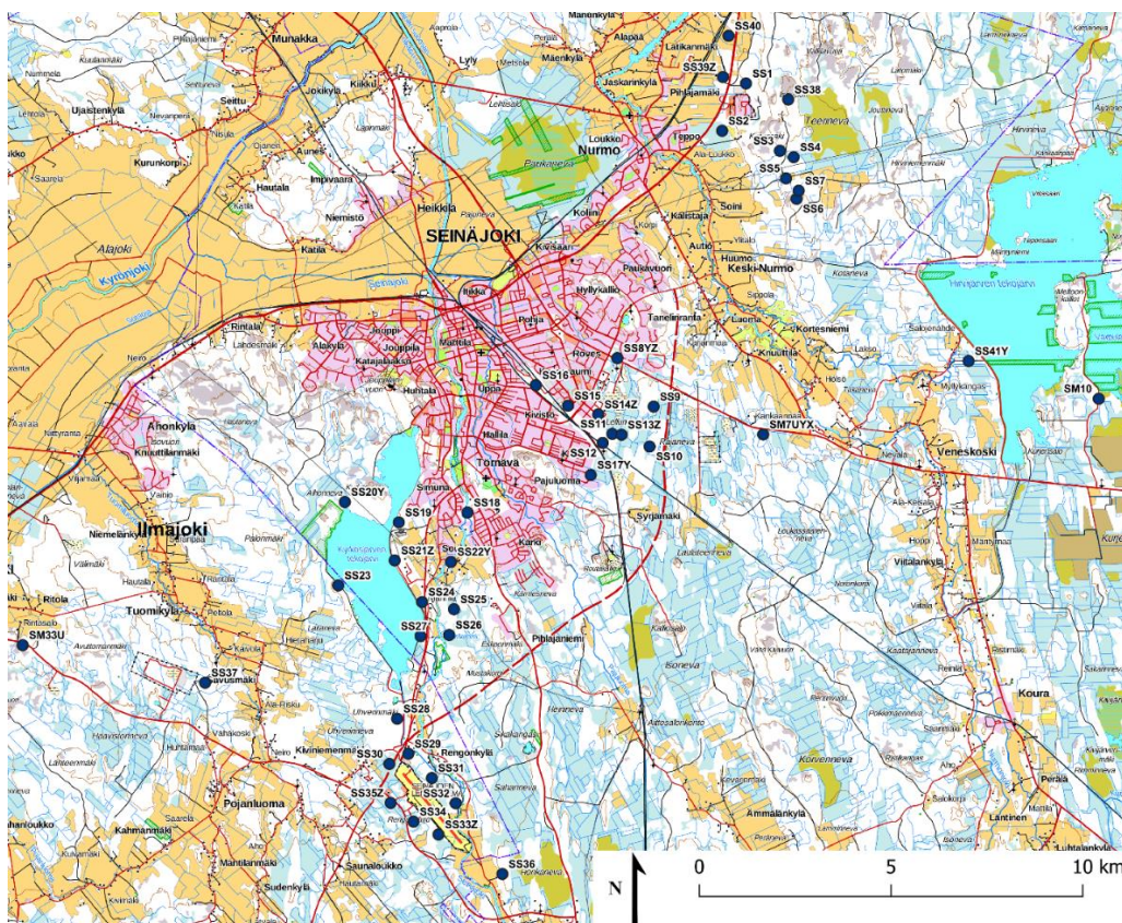
Kuva 3-3 Sammalalojen tarkempi sijainti Seinäjoen seudun bioindikaattoritutkimuksessa vuonna 2022. Taustapitoisuusala ja kaksi pohjoisinta alaa eivät näy karttakuvassa.
