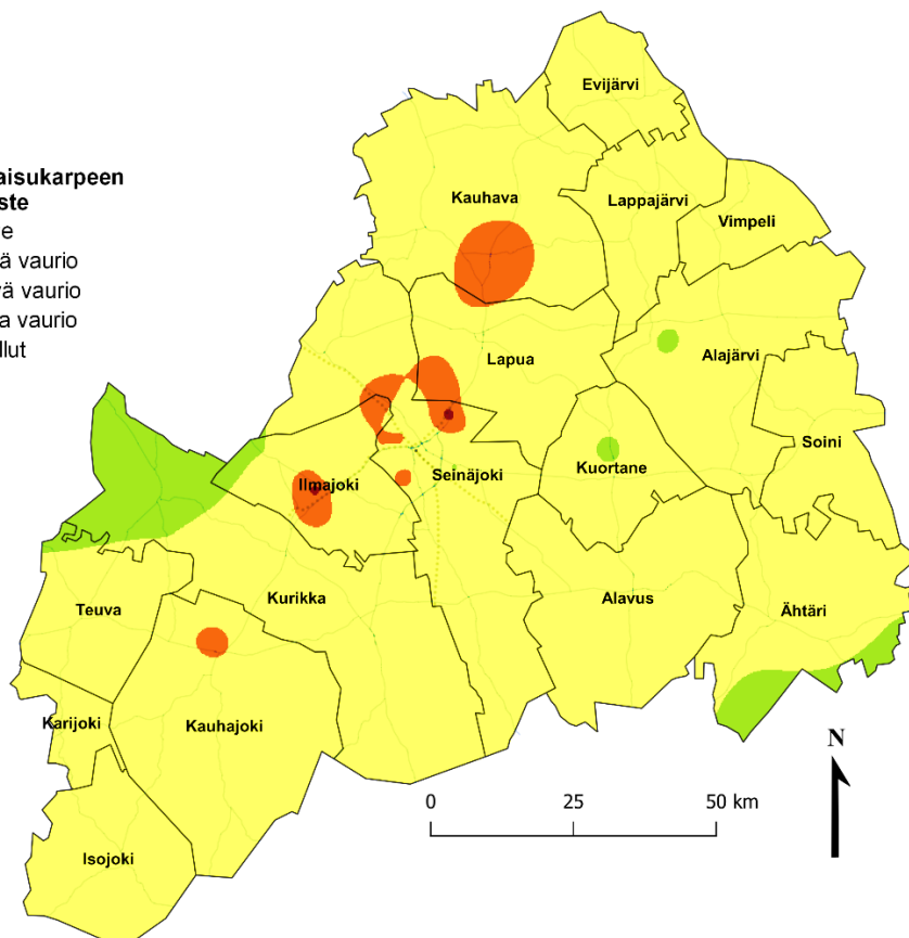
Kuva 4-2. Sormipaisukarpeen vaurioasteen vyöhykkeet tutkimusalueella vuonna 2022.
