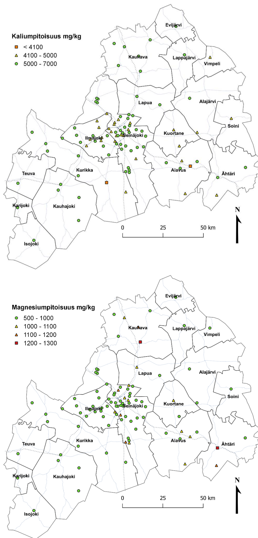
Kuva 4-17. Neulasten kalium- ja magnesiumpitoisuudet tutkimusalueella vuonna 2022.
