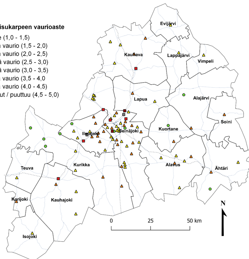
Kuva 4-1. Sormipaisukarpeen vaurioaste tutkimusalueella vuonna 2022.
