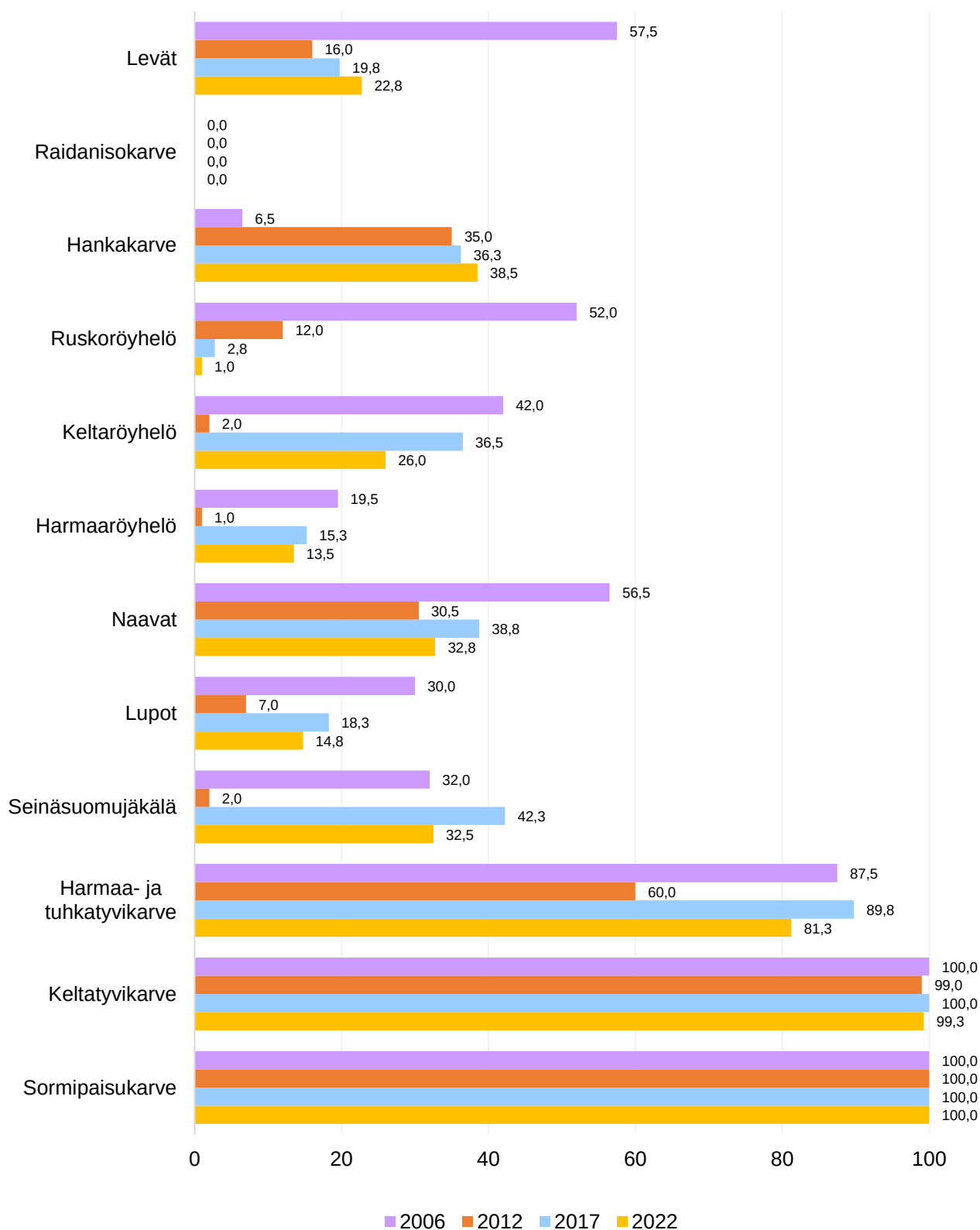
Kuva 5-3. Männyn runkojäkälien prosentuaalinen esiintymistiheys tutkimusrungoilla vuosina 2006 (n = 200, Laita ym. 2008), 2012 (n = 200, Ramboll 2012), 2017 (n = 400, Ahma ympäristö 2017) ja 2022 (n = 400). Vertailussa huomioitu samana pysyneet mäntyhavaintoalat (n = 40).
