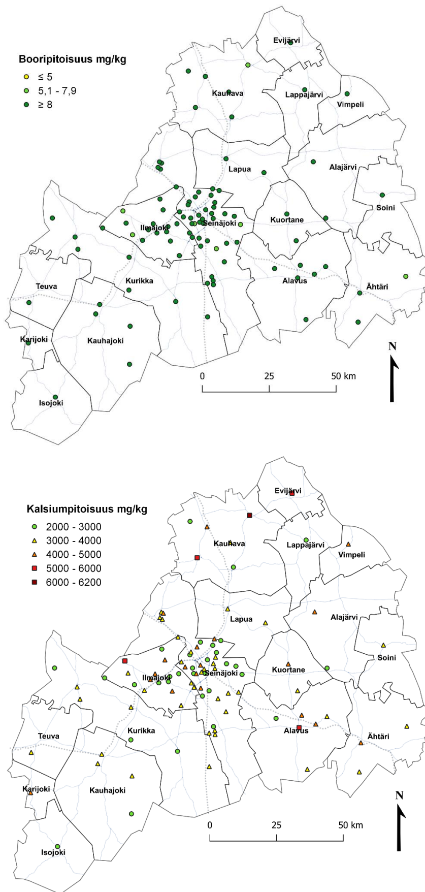
Kuva 4-14. Neulasten boori- ja kalsiumpitoisuudet tutkimusalueella vuonna 2022.
