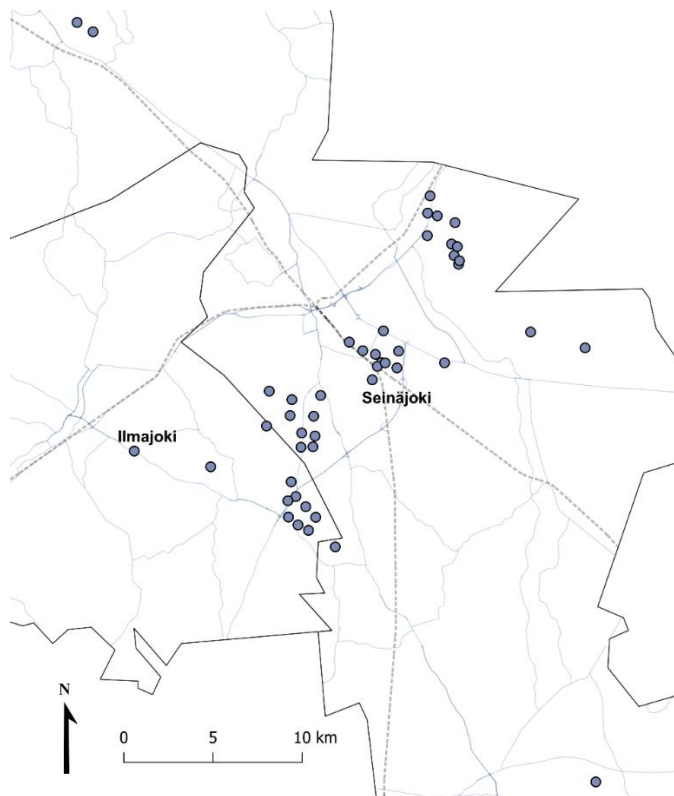
Kuva 3-2 Sammalalat Seinäjoen seudun bioindikaattoritutkimuksessa vuonna 2022 (n = 47).
