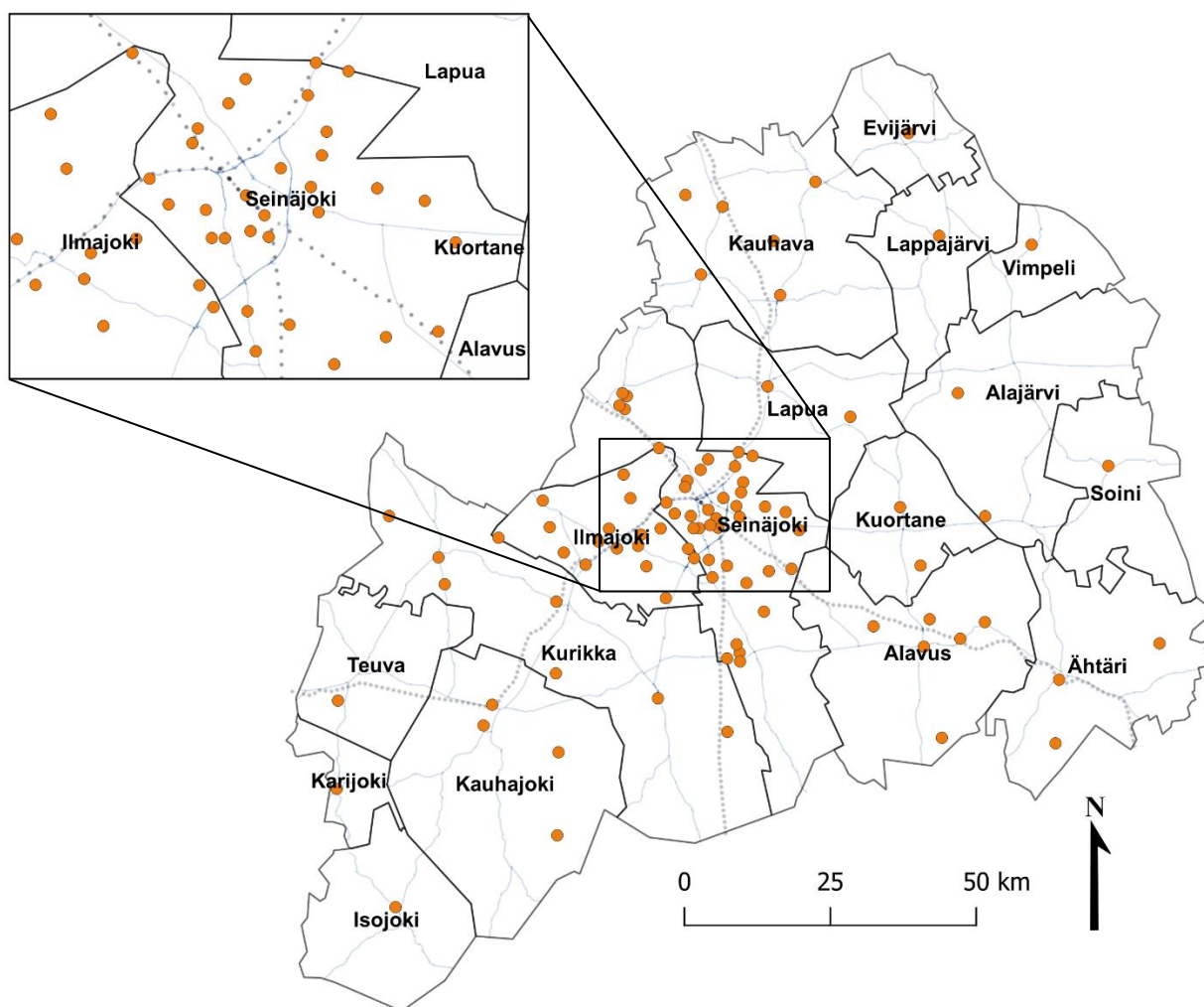
Kuva 3-1 Mäntyhavaintoalat Seinäjoen seudun bioindikaattoritutkimuksessa vuonna 2022 (n = 96).
