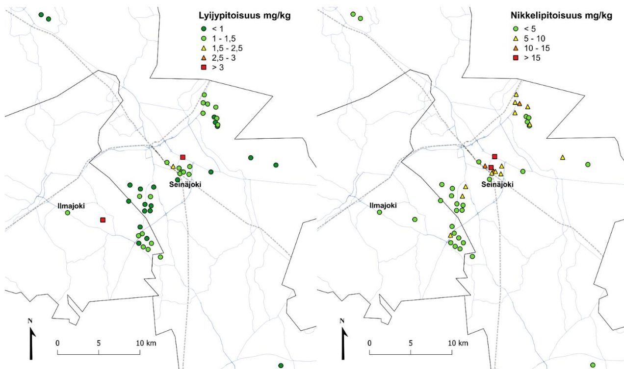
Kuva 4-24. Sammalnäytteiden lyijy- ja nikkelpitoisuus tutkimusalueella heinäkuussa 2022 (n = 47).
