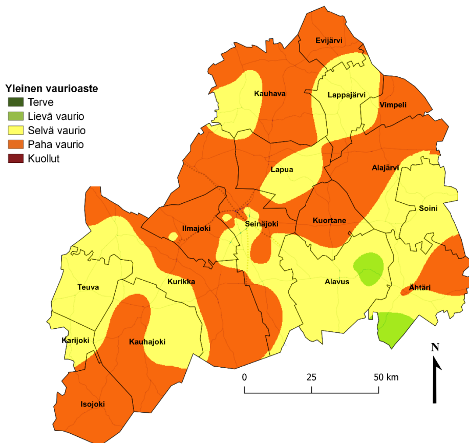
Kuva 4-5. Yleisen vaurioasteen vyöhykkeet tutkimusalueella vuonna 2022.
